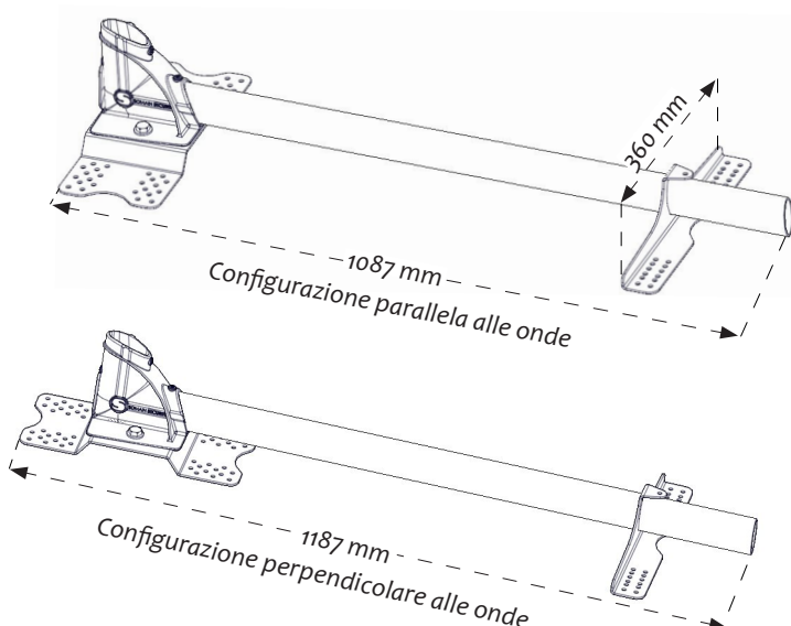
RIF: 100543 Gamba di sostegno.
