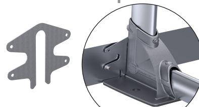
RIF: 100558 Fissaggio del plinto per GCE-BA. Quando l'acroterio è inferiore a 100 mm.
