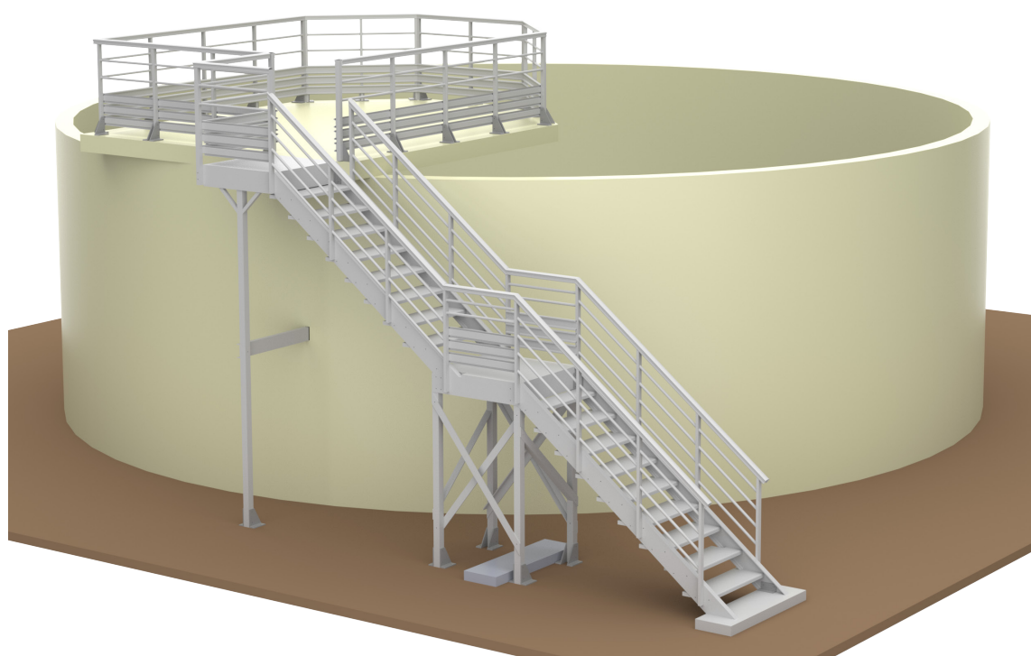
Colocação em conformidade de uma instalação na indústria petroquímica
