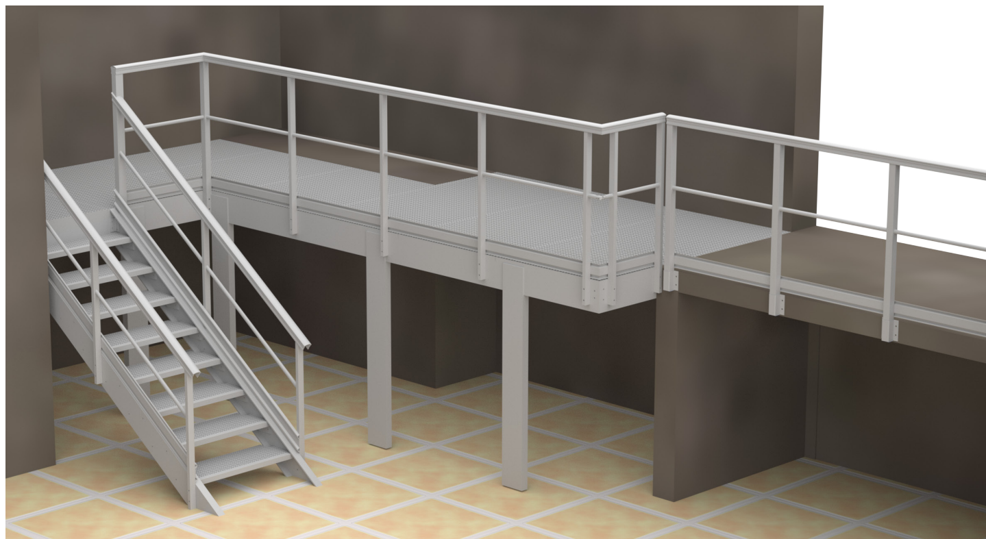
Exemplo de uma instalação completa de compósito que associa escadas, passarela e guarda-corpo.
