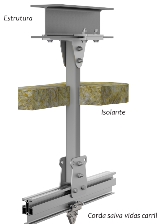
Tubo de isolamento térmico em compósito
